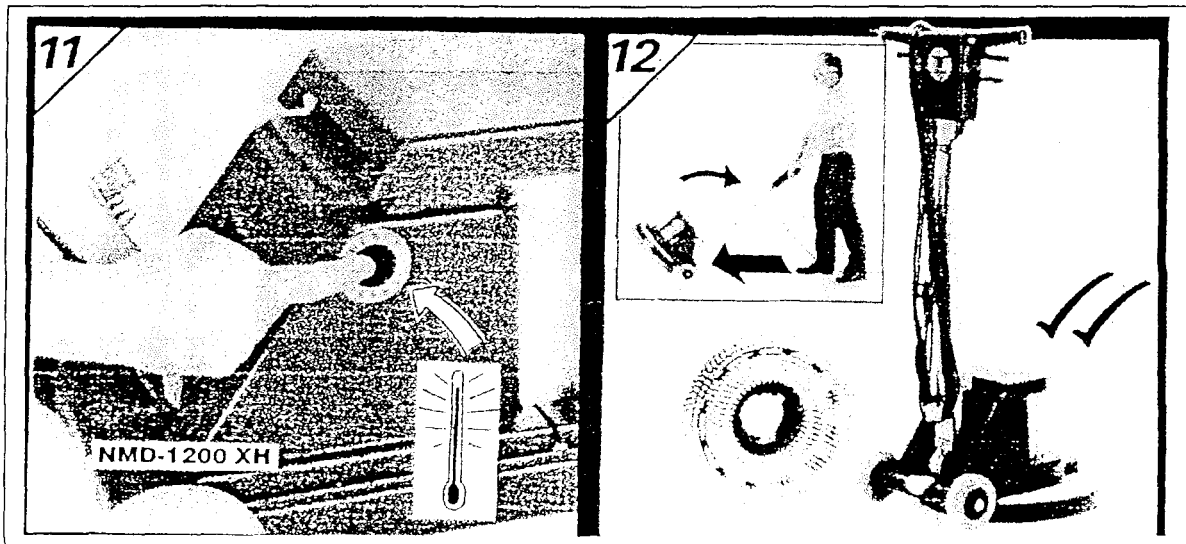
Zabezpieczenie termiczne w urządzeniu 1200 XH, podane zabezpieczenie występuje wyłącznie w modelu 1200 XH, w przypadku przeciążenia silnika zabezpieczenie zadziała wyłączając silnik napędowy, po zadziałaniu zabezpieczenia należy odczekać od 3-4 min w celu ochłodzenia zabezpieczenia
