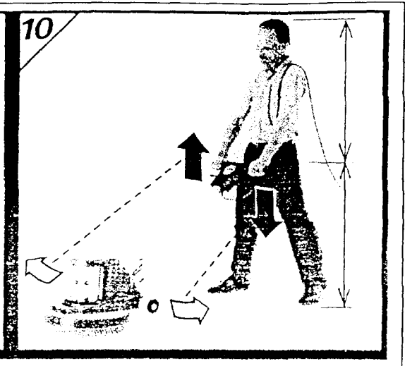
Prawidłowe ustawienie rękojeści w zależności od wzrostu operatora. Zaleca się ustawienie rękojeści na wysokości bioder, zapewnia to maksymalnie komfortową pracę szorowarką
