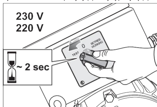
Rys. 77 Silniki jednofazowe: Aby sprawdzić działanie taśmy szlifierskiej, przytrzymaj przycisk przełącznika na silniku w tej pozycji przez ok. 2 sekundy -TEST- przytrzymaj i jednocześnie sprawdź bieg taśmy szlifierskiej. Następnie zwolnij przycisk przełącznika.
