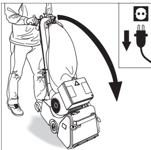
Rys. 96 Wyciągnij wtyczkę z gniazdka i powoli przechyl maszynę do przodu.
