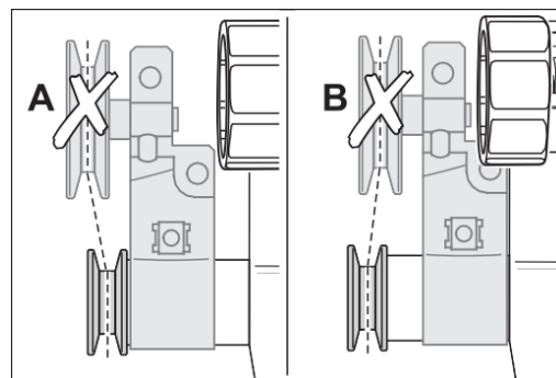
Rys. 113 Unikaj pozycji A i B napinacza paska! W przeciwnym razie może być zwiększone zużycie napinacza paska, wału wentylatora i paska klinowego!
