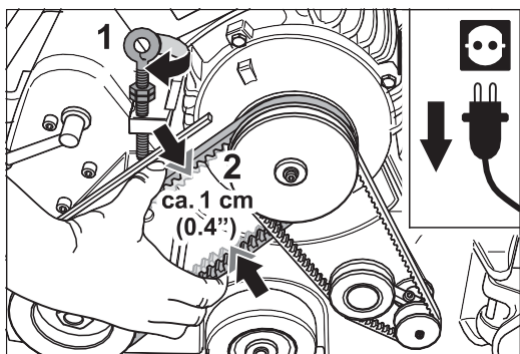
Rys. 110 Aby napiąć pasek napędowy, przekręć śrubę pierścieniową na silniku zgodnie z ruchem wskazówek zegara (1). Prawidłowe napięcie paska napędowego: Pasek klinowy powinien nadal dać się ścisnąć o ok. 1 cm (2).
