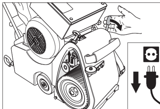
Rys. 40 Nacisnąć dźwignię napinacza w dół. Spowoduje to zaciśnięcie taśmy szlifierskiej.
