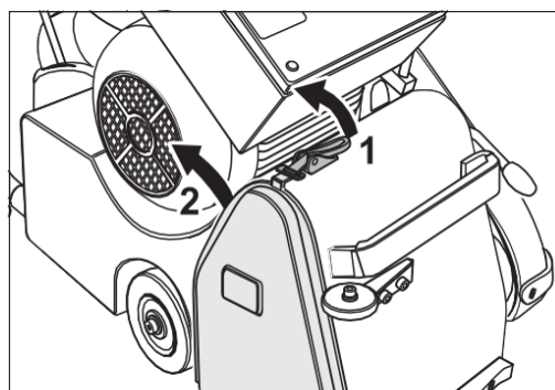
Rys. 76 Otwórz zamek pokrywy (1) i zdejmij pokrywę (2).
