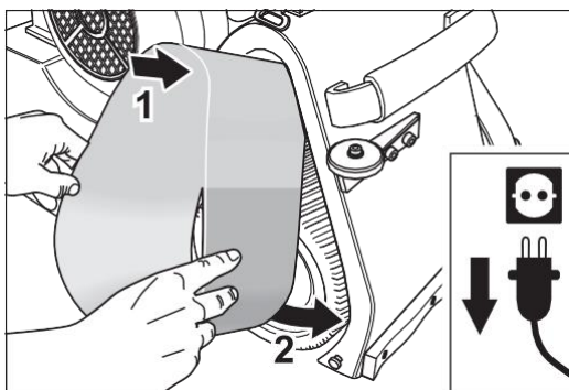
Rys. 15 Umieść taśmę szlifierską na rolce napinającej urządzenia.
