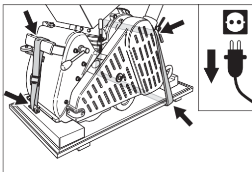
Rys. 46 Transport lub przechowywanie maszyny na dolnej części skrzyni transportowej.
