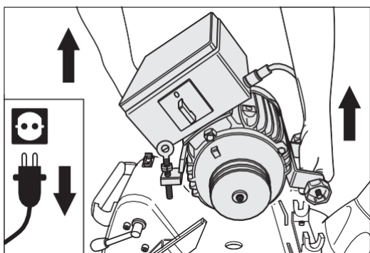
Rys. 54 Wymij silnik z obudowy maszyny.
