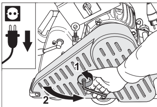
Rys. 102 Wyciągnij wtyczkę z gniazdka i otwórz osłonę paska.
