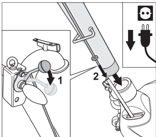
Rys. 8 Podczas wkładania rurki prowadzącej pręt spustowy musi być prawidłowo włożony!
