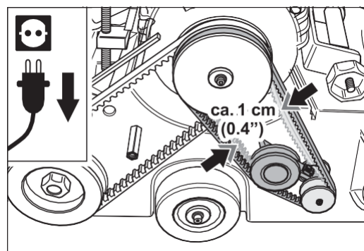
Rys. 115 Prawidłowe napięcie paska: Pasek klinowy powinien nadal dać się ścisnąć o ok. 1 cm.
