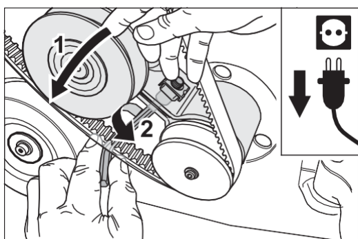
Rys. 114 Aby napiąć pasek klinowy wentylatora, przesuń napinacz paska w lewo (1) i jednocześnie ostrożnie dokręć śrubę zaciskową (2).
