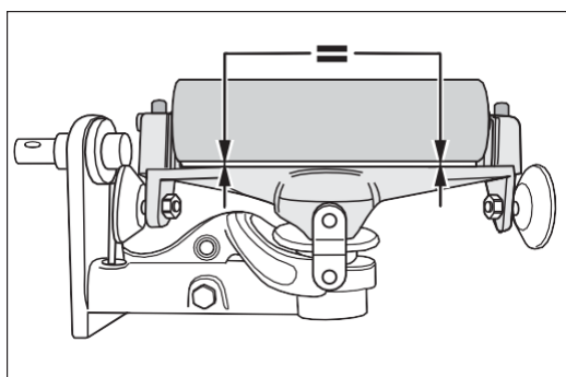
Rys. 94 ... wałek napinający leżał równoległa do górnej części urządzenia .
