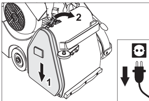
Rys. 41 Po pomyślnym sprawdzeniu i ustawieniu biegu taśmy szlifierskiej ponownie załóż pokrywę komory papieru.
