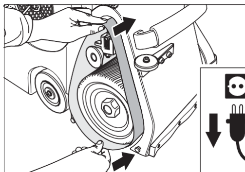
Rys. 16 Przesunij taśmę szlifierską na rolkę napinającą i rolkę szlifierską.
