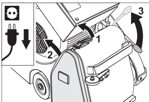
Rys. 87 Otwórz zamek pokrywy (1) i zdejmij pokrywę (2). Pociągnij do góry dźwignię napinacza na urządzeniu (3) i tym samym opuść wałek napinający.
