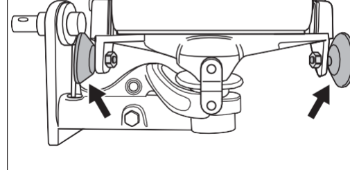
Abb. 73 Die beiden Leitrollen müssen leicht drehbar sein! Schwergängige oder feststehende Leitrollen müssen ersetzt werden (Brandgefahr)!
