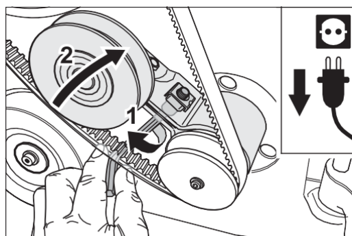
Rys. 106 Poluzuj śrubę zaciskową napinacza paska (1) i poluzuj pasek klinowy (2).
