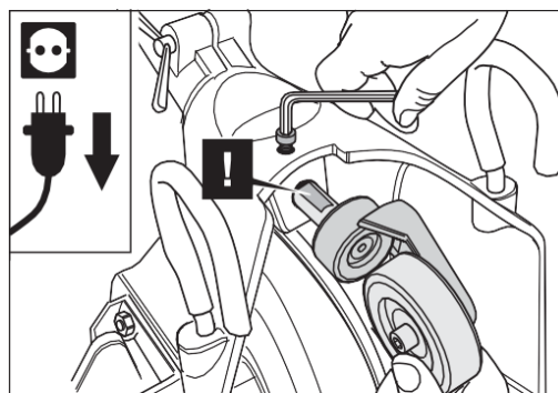
Abb. 99 Poluzuj śrubę mocującą i wyciągnij całe tylne koło z obudowy maszyny. Podczas montażu wyrównaj powierzchnię zaciskową osi w kierunku śruby.
