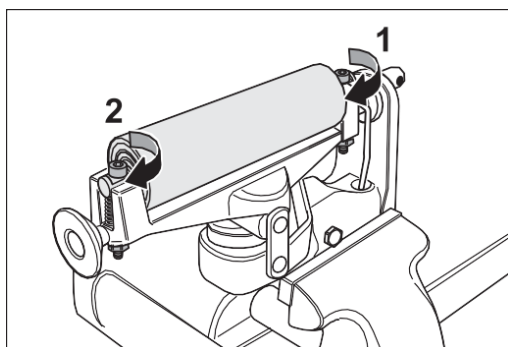
Rys. 93 Najpierw dokręć śrubę po stronie nieresorowanej (1), a następnie po stronie sprężynowej (2), aby...
