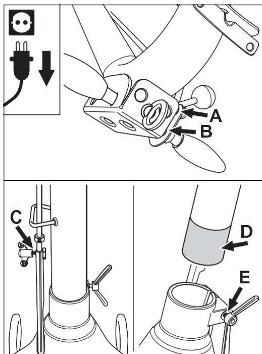
Rys. 74 Punkty smarowania, które należy regularnie oliwić.
