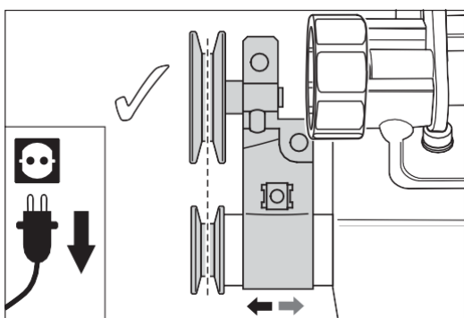
Rys. 112 Rowki paska klinowego napinacza paska i osi wentylatora muszą być ustawione w jednej linii! Przesuń odpowiednio napinacz paska.
