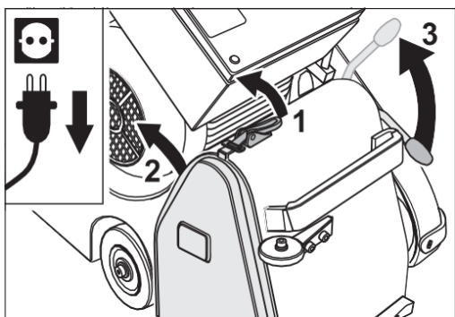
Rys. 35 Otwórz blokadę pokrwyty (1) i zdejmij pokrwyte (2). Pociągnij do góry dźwignię napinacza (3) i tym samym opuść wałek napinający.
