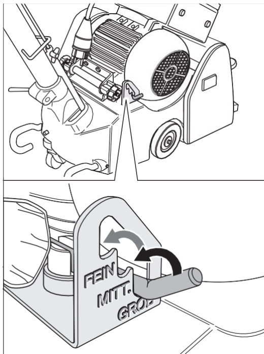
Rys. 33 Różne poziomy nacisku szlifowania można ustawić za pomocą dźwigni regulacyjnej.
