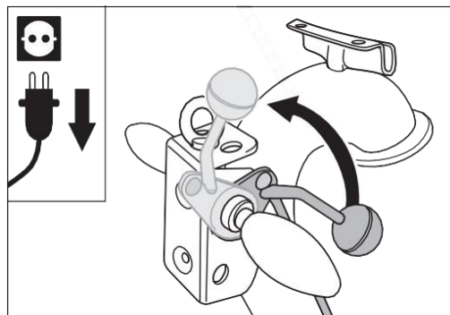
Rys. 11 Pociągnij do góry dźwignię spustu na uchwycie do oporu. To podnosi bęben szlifierski z ziemi.
