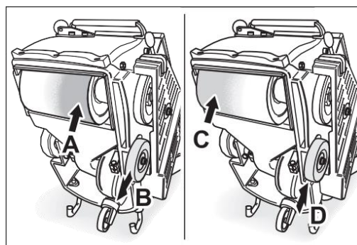
Rys. 84 Jeśli maszyna szlifuje mocniej po stronie A, koło należy wyregulować w kierunku B. Jeśli maszyna szlifuje więcej po stronie C, koło należy wyregulować w kierunku D.
