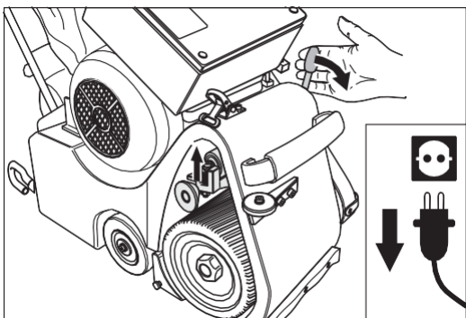
Rys. 69 Nacisnąć dźwignię obsługową urządzenia w dół. Spowoduje to podniesienie wałka napinającego.
