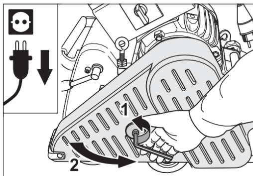
Rys. 2 Wyciągnij wtyczkę z gniazdka i otwórz osłonę paska.
