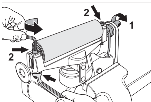
Rys. 91 Ustaw górną część urządzenia w najwyższej pozycji (1). Odkręć dwie śruby mocujące wałka napinającego i jednocześnie przytrzymaj nakrętki zabezpieczające kluczem oczkowym (2).
