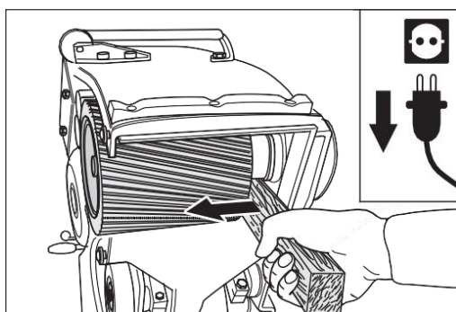
Rys. 90 Jeśli wałek szlifujący jest zablokowany, użyj drewnianej dźwigni. Nie używaj siły!
