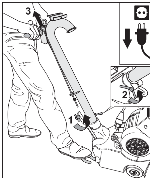
Rys. 56 Odkręcić śrubę motylkową na dyszlu podnoszącym (1) i nakrętkę motylkową na obudowie maszyny (2). Następnie wyciągnij rurę prowadzącą z obudowy maszyny (3).
