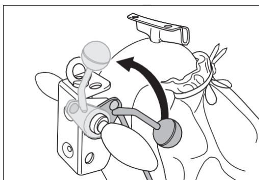
Rys. 34 Pociągnij do góry dźwignię hebla na uchwycie do oporu. To podnosi wałek szlifierski z podłogi.
