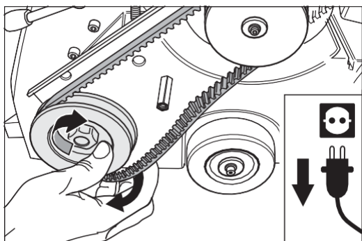
Rys. 108 Zsuń pasek napędowy dolnego koła pasowego. W razie potrzeby użyj klucza rolkowego (patrz torba z narzędziami). Ale klucz do cylindrów obracaj tylko zgodnie z ruchem wskazówek zegara, aby nie poluzować nakrętki!
