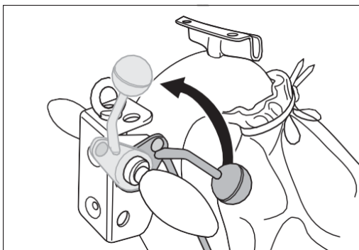
Rys. 95 Pociągnij do góry dźwignię spustową na uchwycie do oporu. To podnosi wałek szlifujący z podłogi.
