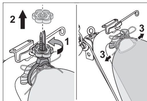
Rys. 44 Poluzuj MultiClip (1 i 2) i otwórz pętlę na worku na pył (3).
