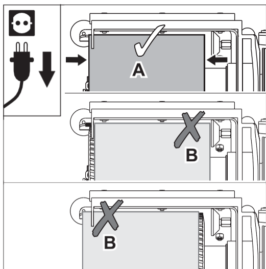
Rys. 17 Nasuń taśmę szlifierską na wałek napinający i wałek szlifujący, aż wałek szlifujący zostanie równomiernie pokryty z obu stron przez taśmę szlifierską (A).
