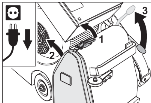
Rys. 14 Otwórz zamek pokrywy (1) i zdejmij pokrywę (2). Pociągnij do góry dźwignię napinacza na urządzeniu (3) i tym samym opuść rolkę napinającą.
