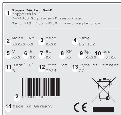
Rys. 7 Informacje na tabliczce znamionowej silnika (patrz tekst główny).
